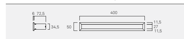
D0005 Difusor de entrada de ar dupla
