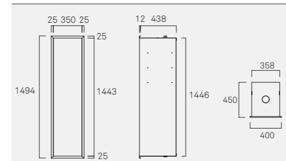
C1000 Porta-lenha.
