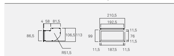
D0002 Difusor de entrada de ar simples
