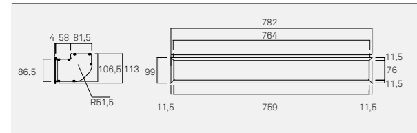
D0015 Difusor de entrada de ar quádrupla
