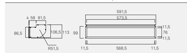
D0015 Difusor de entrada de ar quádrupla
