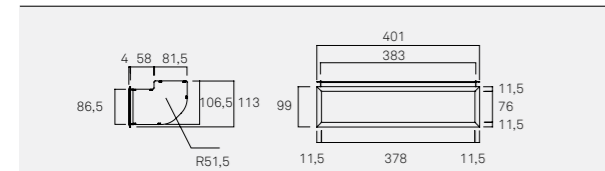
D0007 Difusor de entrada de ar dupla
