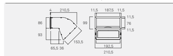
D1002 Difusor de saída de ar simples
