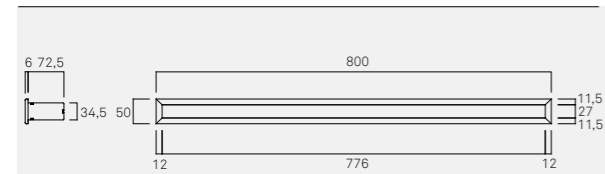
D0010 Difusor de entrada de ar tripla
