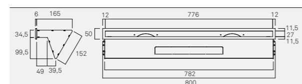
D1010 Difusor de saída de ar tripla
