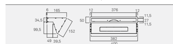
D1005 Difusor de saída de ar dupla
