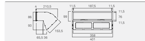
D1007 Difusor de saída de ar simples
