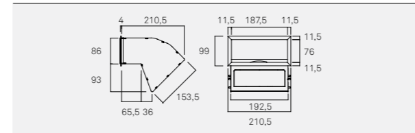
D1002 Difusor de saída de ar simples estreito
