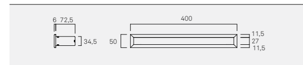
D0005 Difusor de entrada de ar dupla
