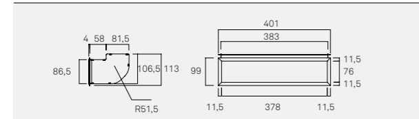
D0007 Difusor de entrada de ar dupla estreito
