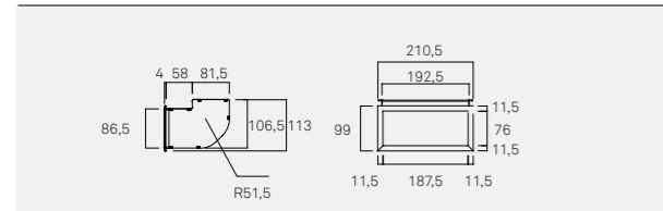
D0002 Difusor de entrada de ar estreito
