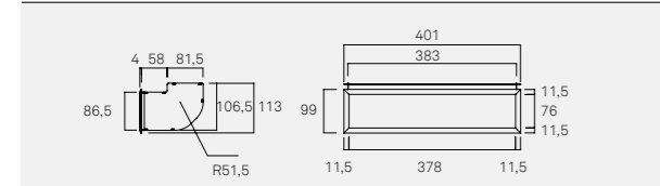
D0007 Presa d'aria doppia stretto
