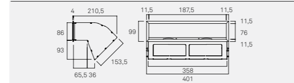
D1007 Diffusore uscita d'aria singolo stretto
