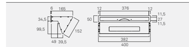
D1005 Diffusore uscita d'aria doppio
