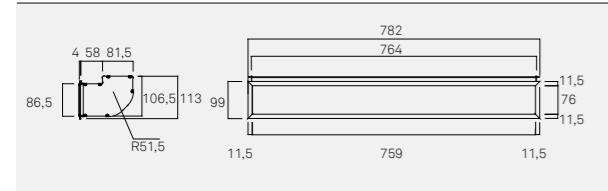
D0015 Presa d'aria quadrupla
