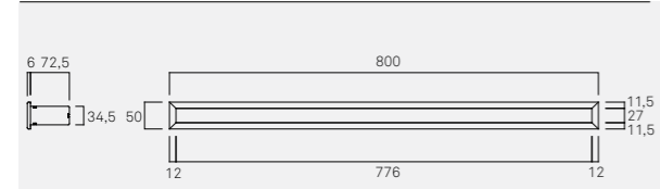
D0010 Presa d'aria tripla
