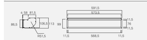
D0015 Presa d'aria quadrupla
