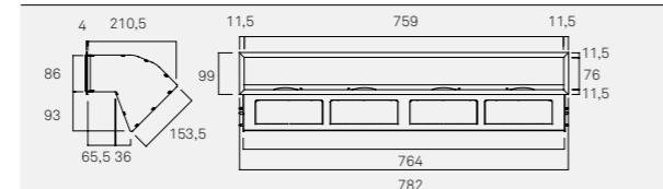
D1015 Diffusore uscita d'aria quadruplo
