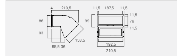
D1002 Diffusore uscita d'aria singolo stretto
