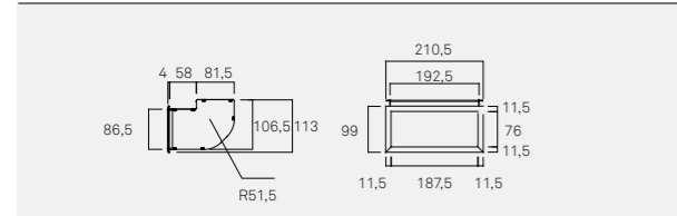
D0002 Presa d'aria singola stretto
