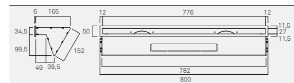
D1010 Diffusore uscita d'aria triplo
