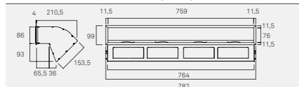
D1015 Difusor de saída de ar quádrupla
