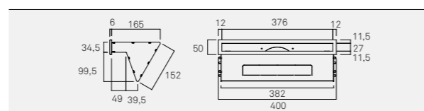
D1005 Difusor de saída de ar dupla
