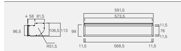
D0015 Difusor de entrada de ar quádrupla
