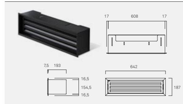
D0000 Difusor de entrada de ar simples
