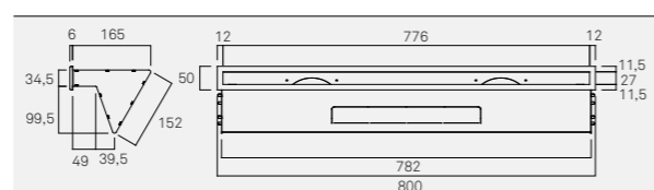
D1010 Difusor de saída de ar tripla
