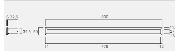
D0010 Difusor de entrada de ar tripla
