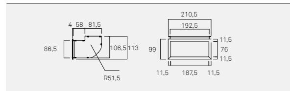
D0002 Difusor de entrada de ar simples
