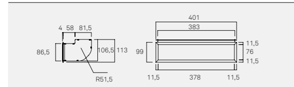
D0007 Difusor de entrada de ar dupla
